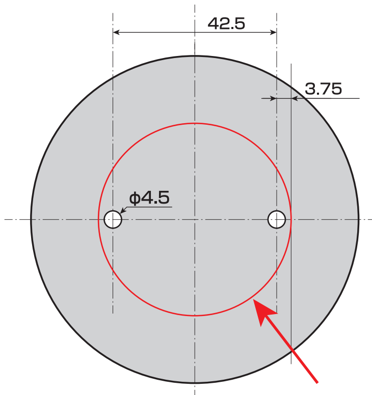
φ85台座
